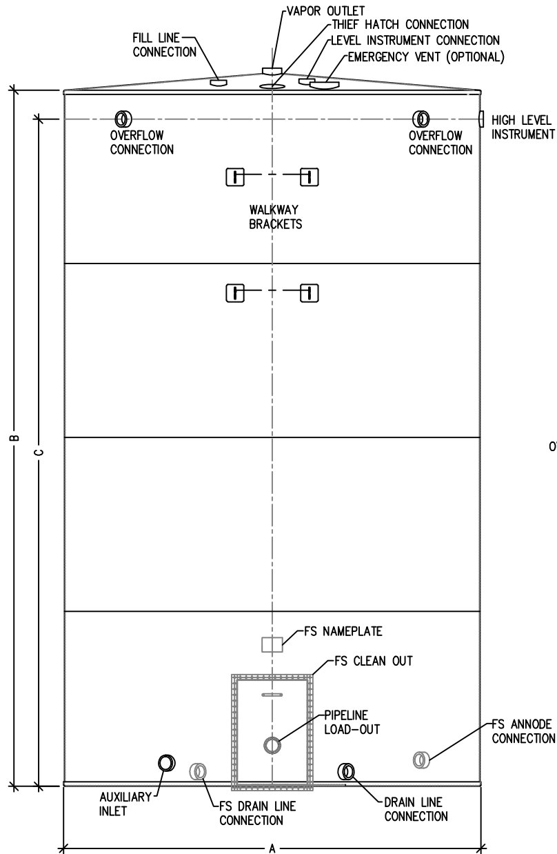
ELEVATION
